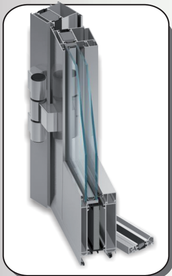
MB 70 drzwi
