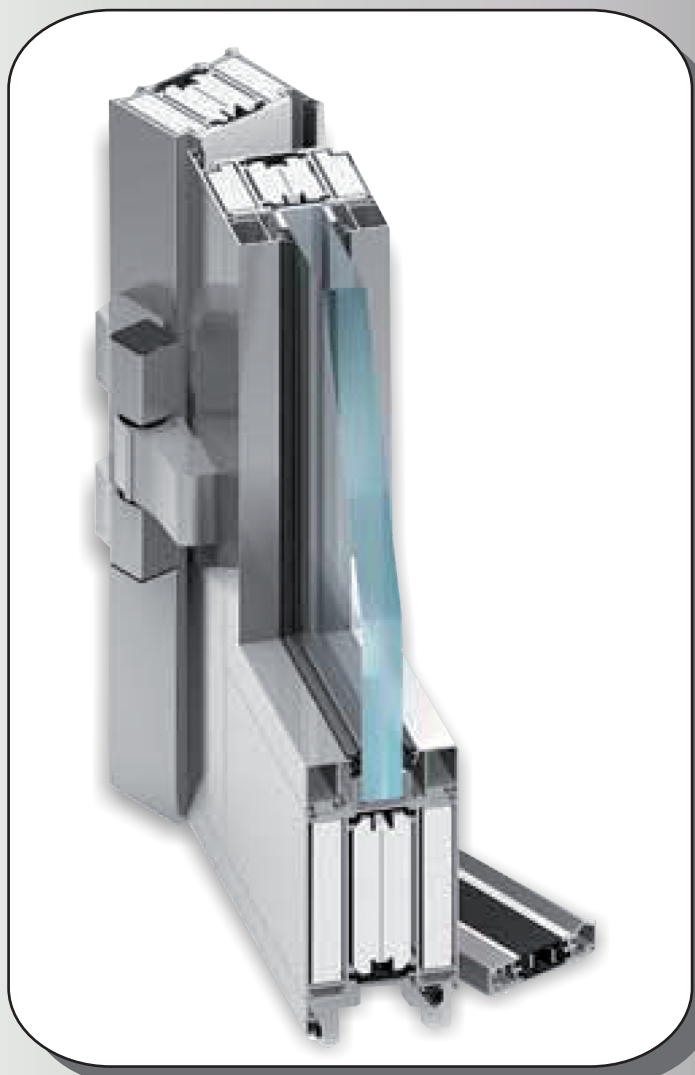
MB 78 EI
